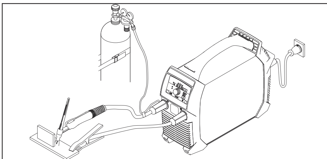
Zavarivanje TIG postupkom, gorionik za zavarivanje s ventilom za blokiranje plina
